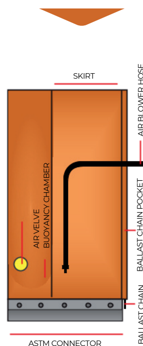
بوم مهار آلودگی نفتی بادشونده
